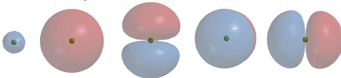
Bild 1: Einfache Wellenfunktionen des Wasserstoffatoms (Quelle http://commons.wikimedia.org/wiki/File:AOS-3D-dots.png , Benjah-bmm27 )
