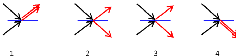
Bild 2: Prinzip des Hong-Ou-Mandel-Effekts: Die vier Möglichkeiten für zwei Photonen an einem Strahlteiler
